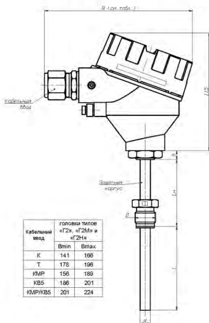
ТС (ТС.К, ТС.П) с головками типов «Г2»: Г2/Exd, Г2/Exd «Г2Н»: Г2Н/Exd, Г2Н/Exd «Г2М»: Г2М/Exd, Г2М/Exd (материал головок типов «Г2» и «Г2М» - алюминиевый сплав, материал головки типа «Г2Н» - нержавеющая сталь)
