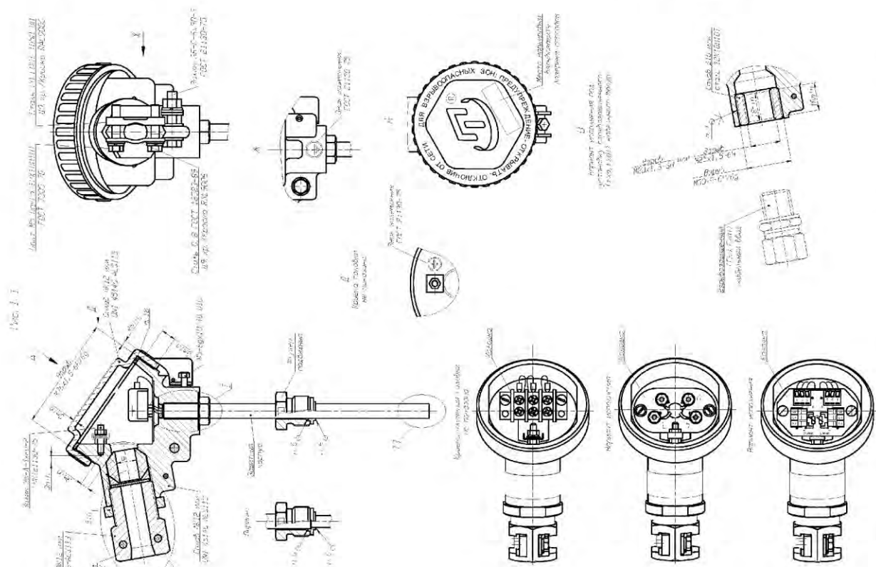
Рисунок 1.1 - Чертеж средств взрывозащиты исполнений ТС (ТС.К, ТС.П)-Exd (Exd) моделей ТСМ (ТСП) 012 (012.К, 012.П) с головкой типа "Г1"
